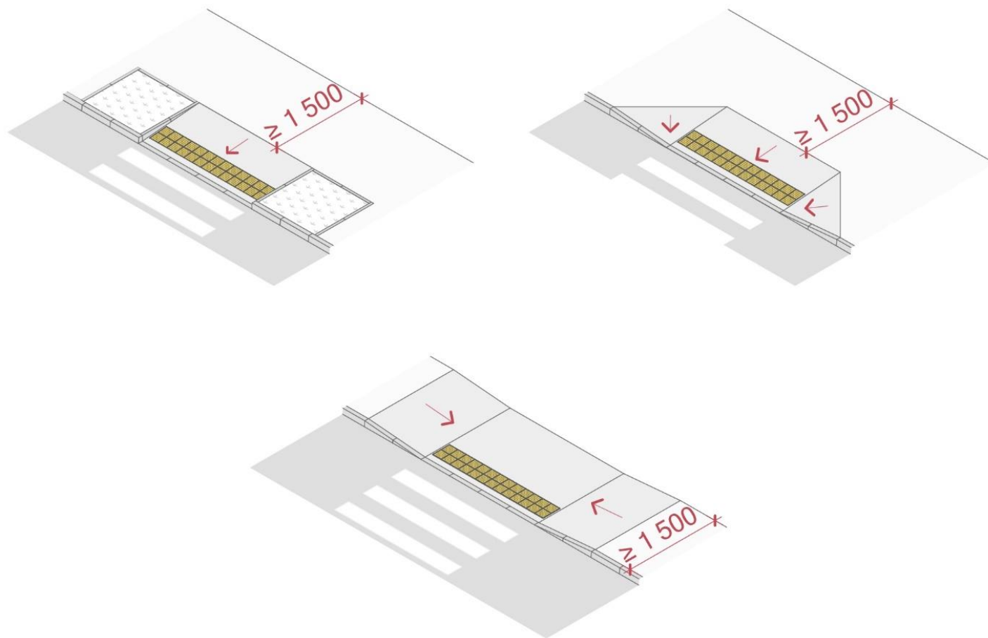
Рис. 7 Приклад облаштування бордюрного пандусу (пониження від тротуару до проїзної частини)
