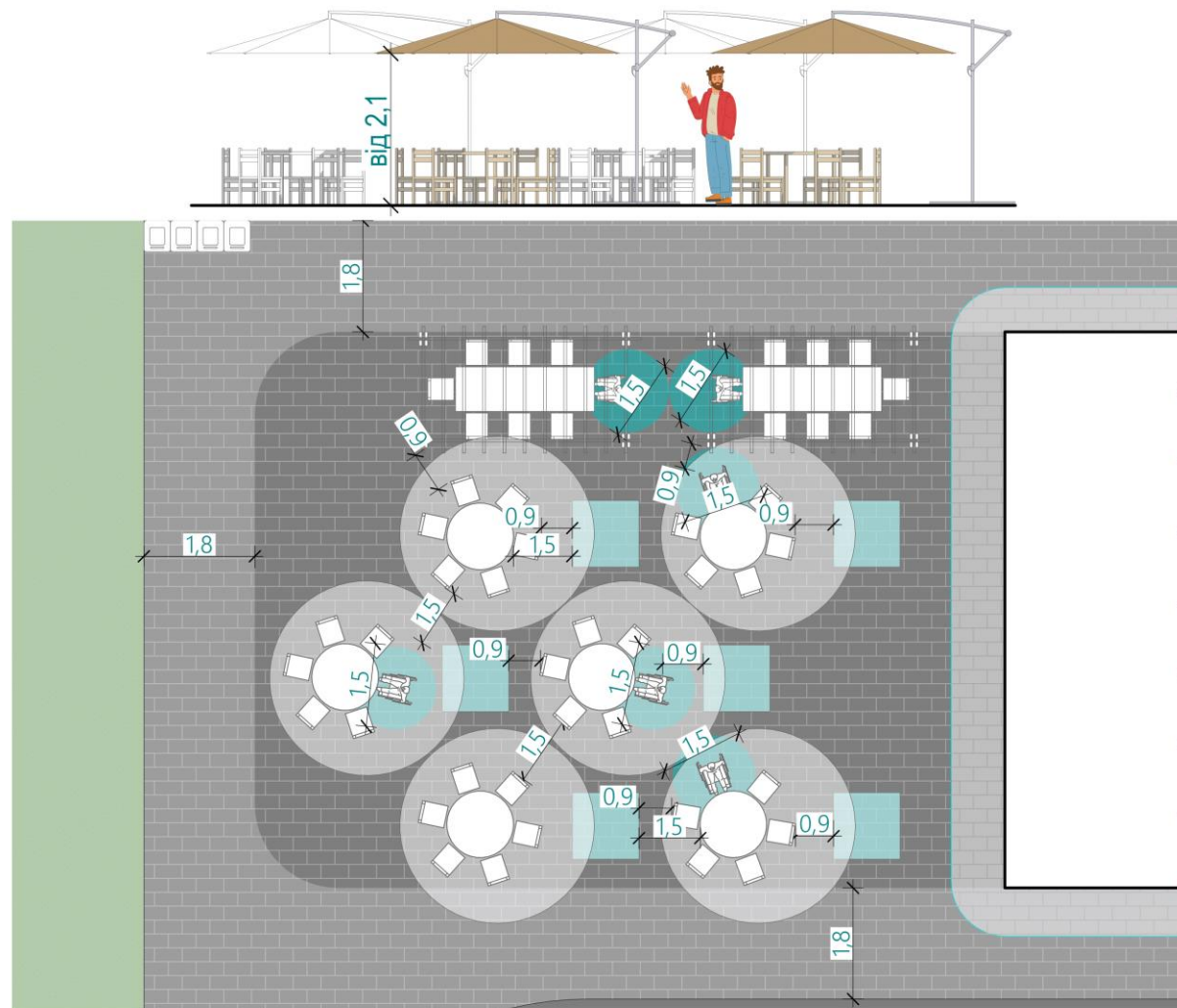
Рис. 13 Орієнтовна схема влаштування відкритого майданчика для відпочинку та прийому їжі.
