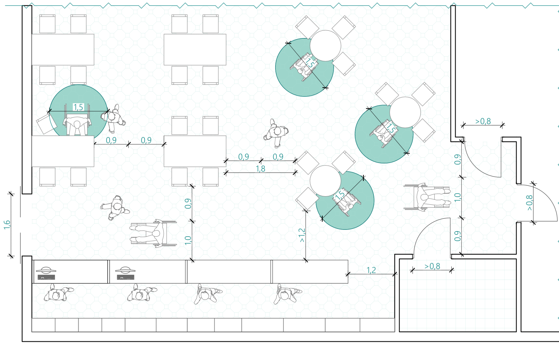
Рис. 22 Орієнтовна схема залу зон для відпочинку та прийому їжі.
