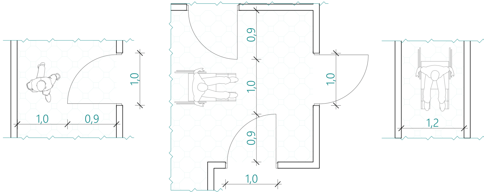
Рис. 21 Габарити коридорів при різному відкриванні дверей.
