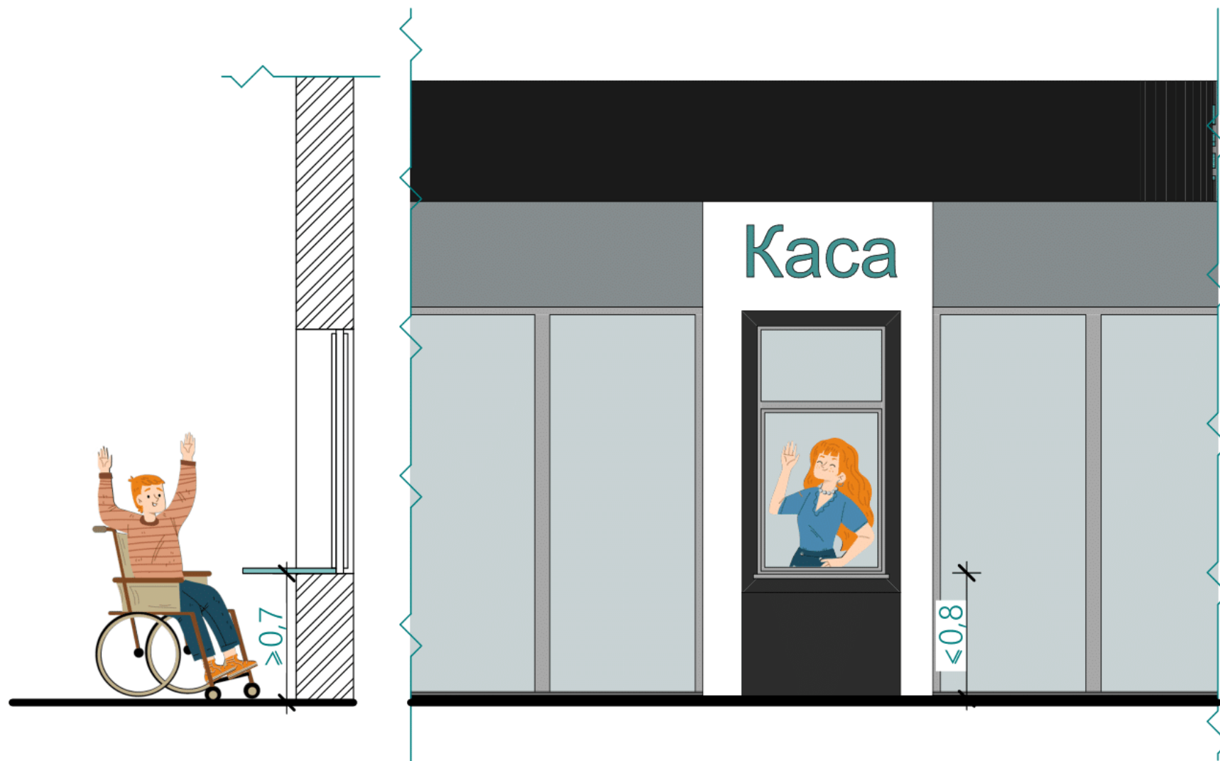
Рис. 16 Схема влаштування касового вікна.
