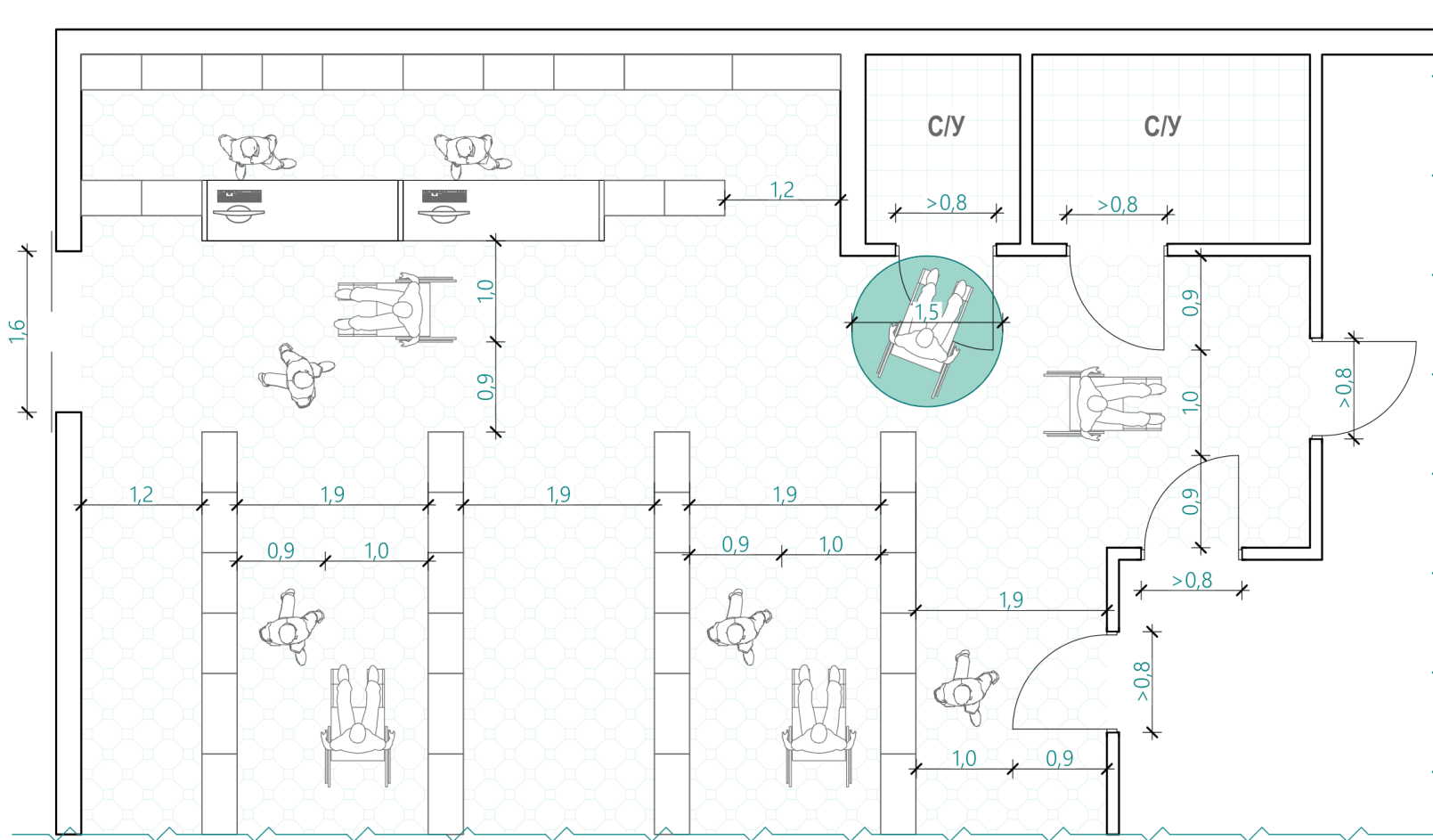
Рис. 20 Орієнтовна схема торгової зали у приміщенні АЗК.
