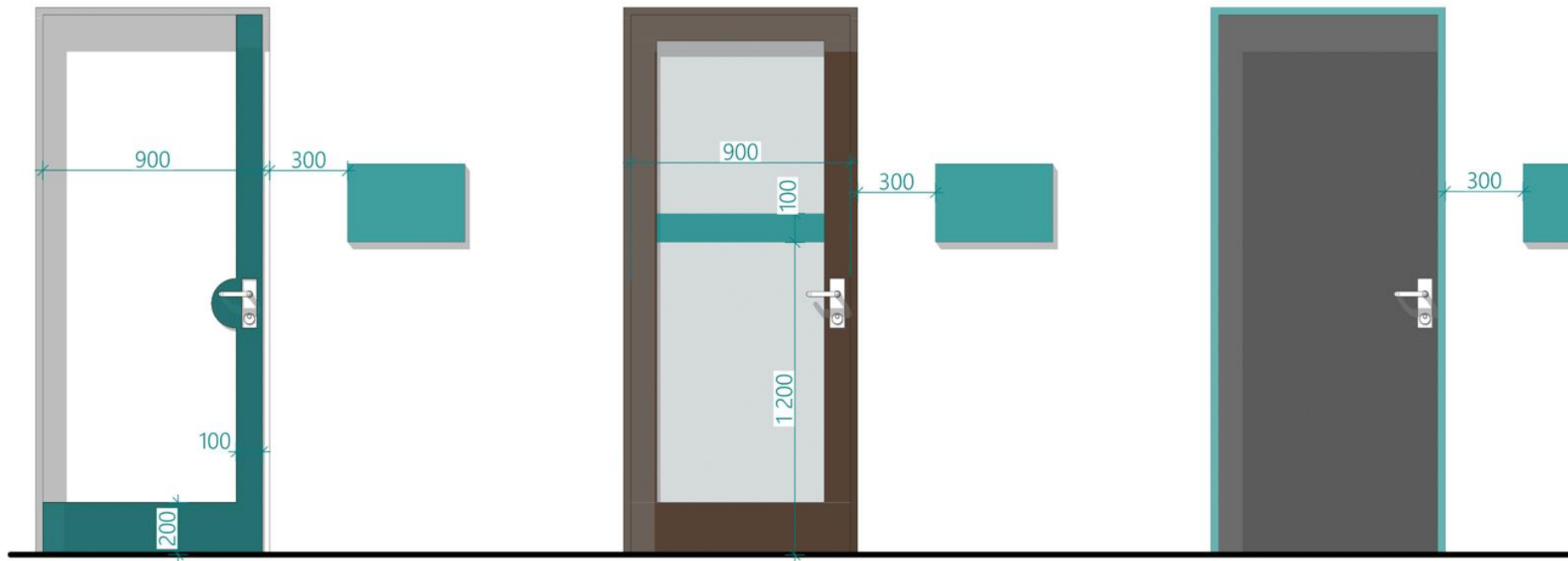
Рис. 32 Контрастне маркування дверей всередині об'єкта.
