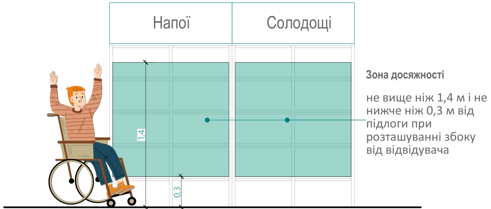
Рис. 18 Схема обладнання торгових площ при боковому підході.
