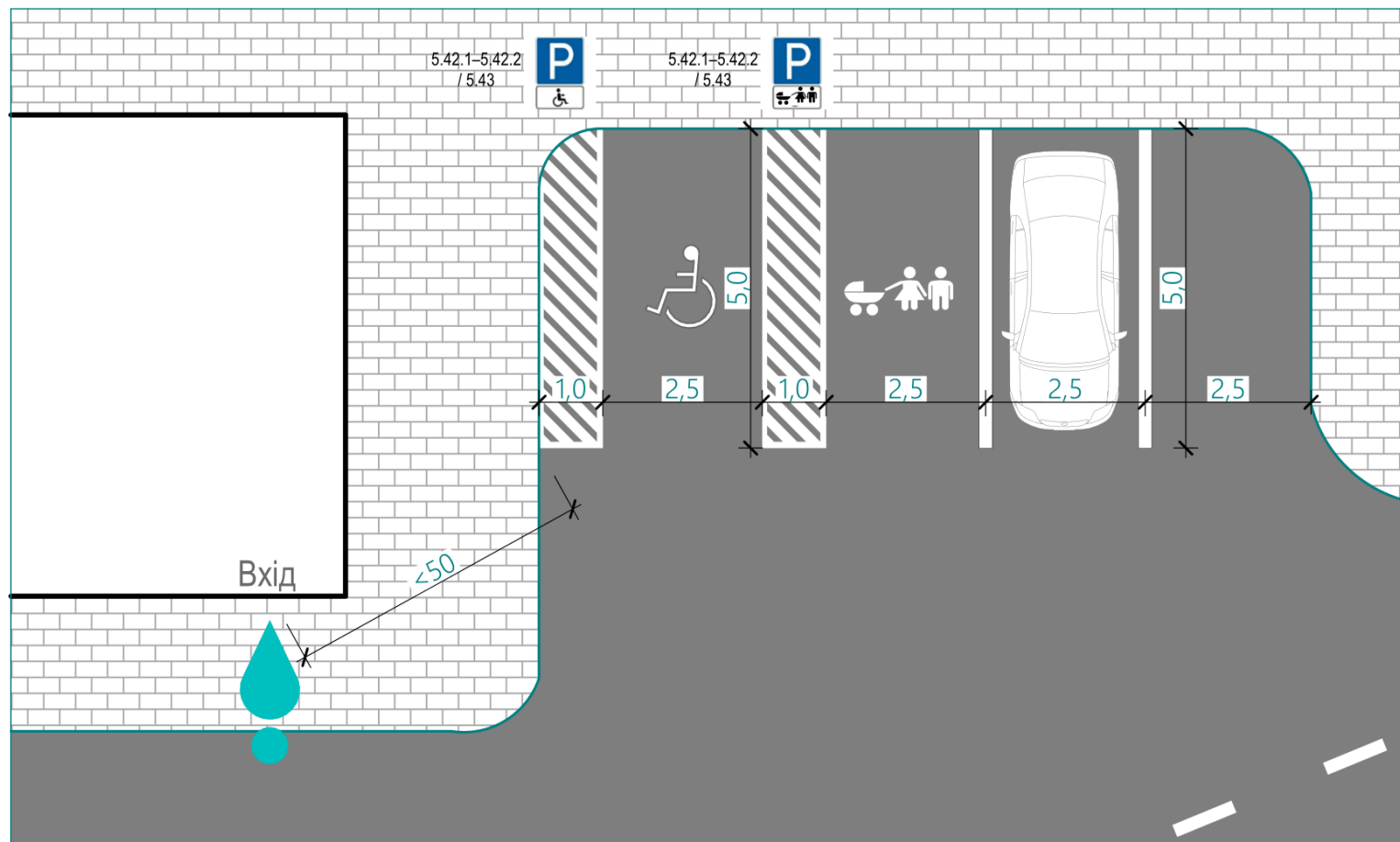
Рис. 10 Схема влаштування паркомісць.
