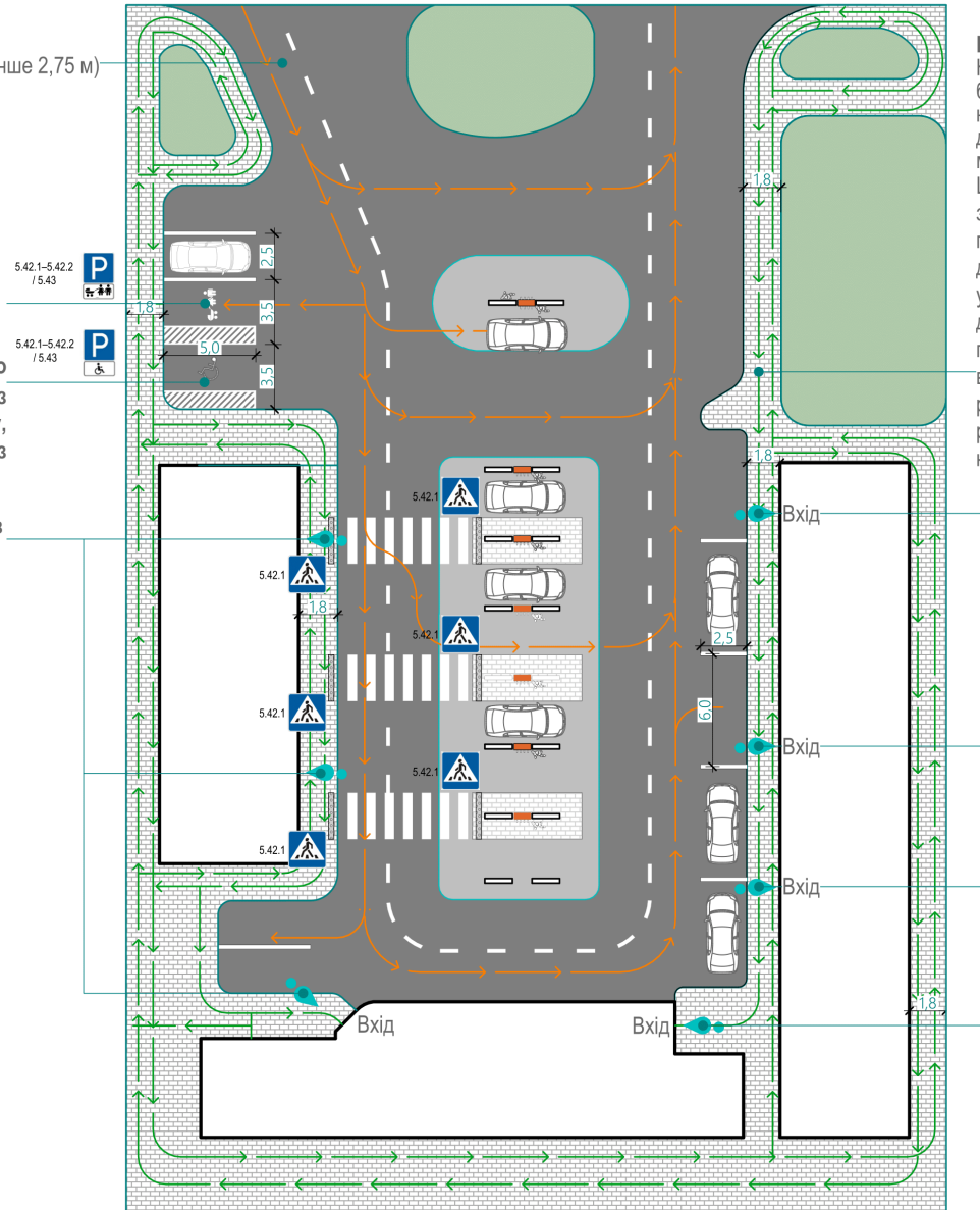
Рис. 8 Схема пішохідного шляху користувача до об'єктів надання послуг.
