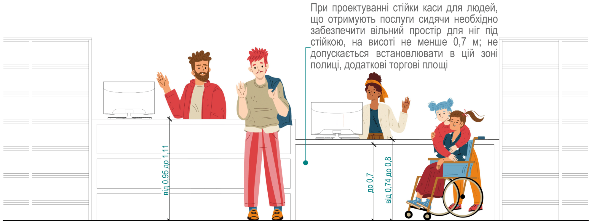
Рис. 17 Схема каси.
