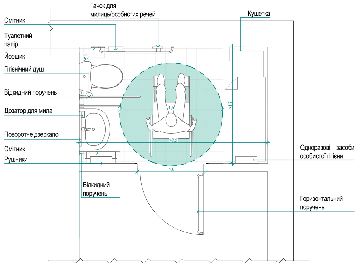
Рис. 27 Орієнтовна схема облаштування універсального санітарного приміщення.
