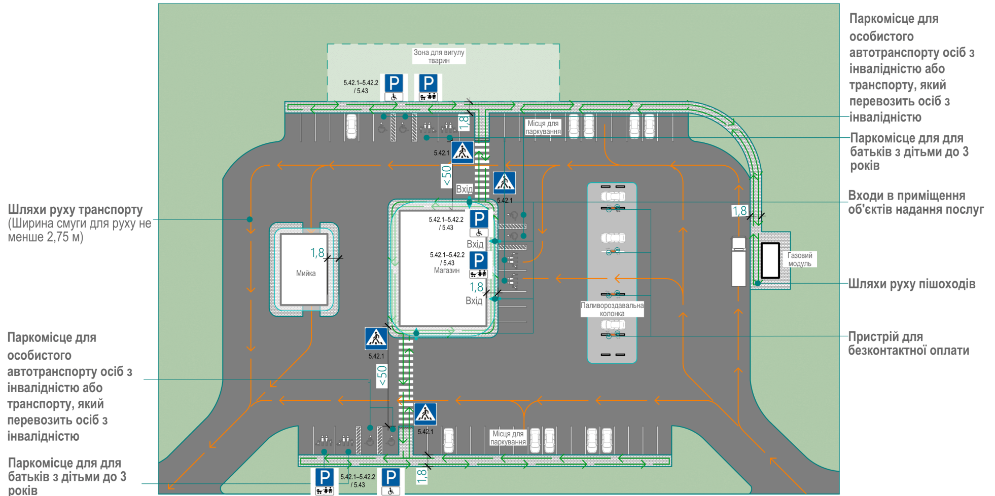
Рис. 9 Схема пішохідного шляху користувача до об'єктів надання послуг.
