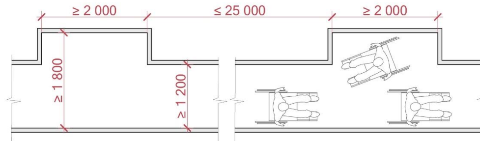
Рис. 2 Приклад облаштування пішохідної доріжки з роз'їзними карманами.
