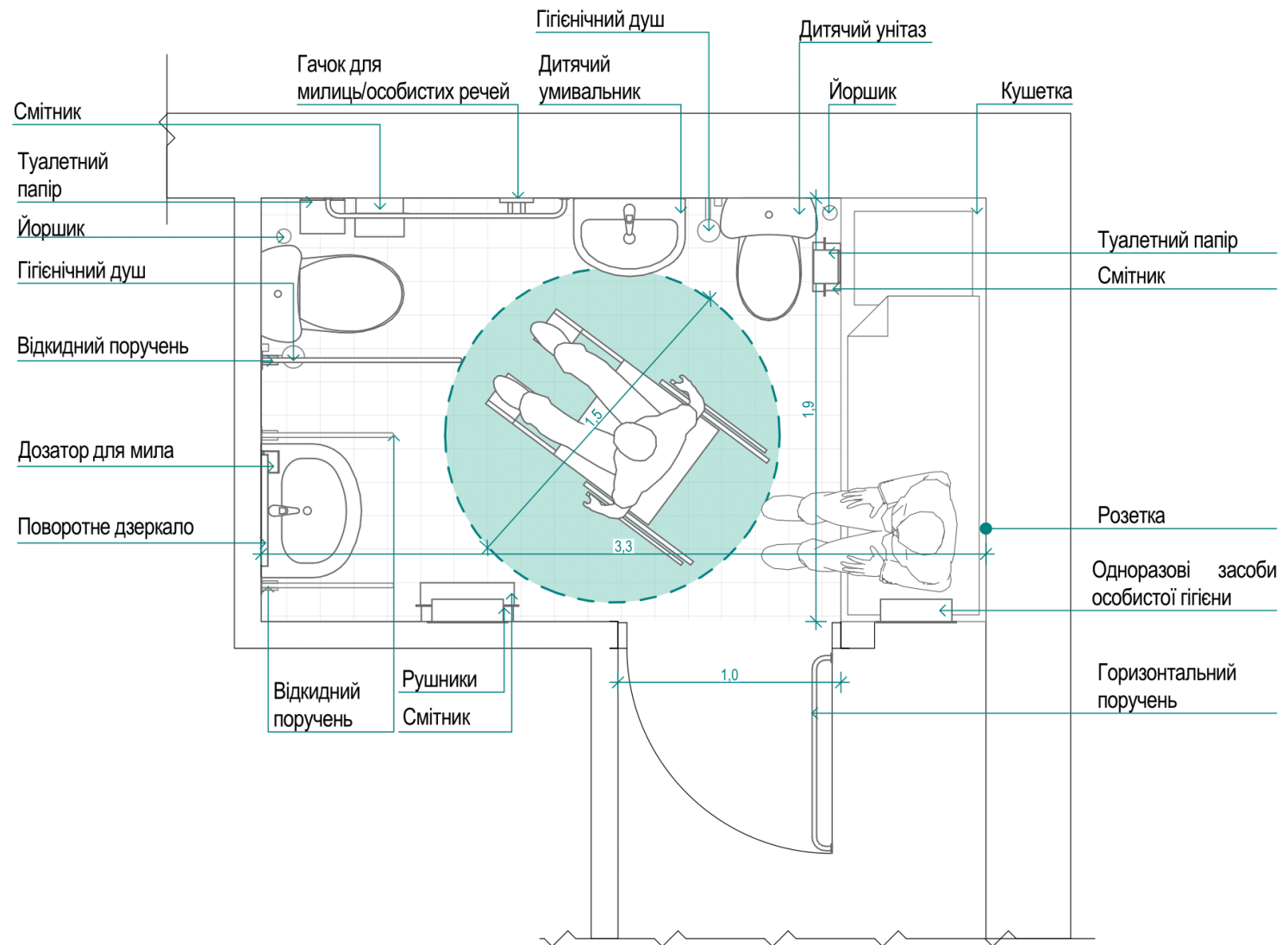
Рис. 28 Орієнтовна схема облаштування сімейного універсального санітарного приміщення.
