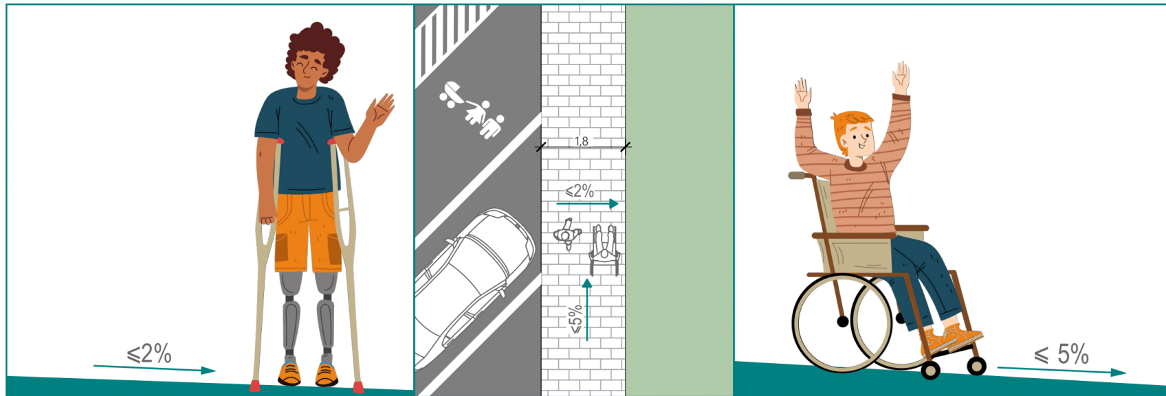
Рис. 5 Поперечний та повздовжній похили пішохідних доріжок.
