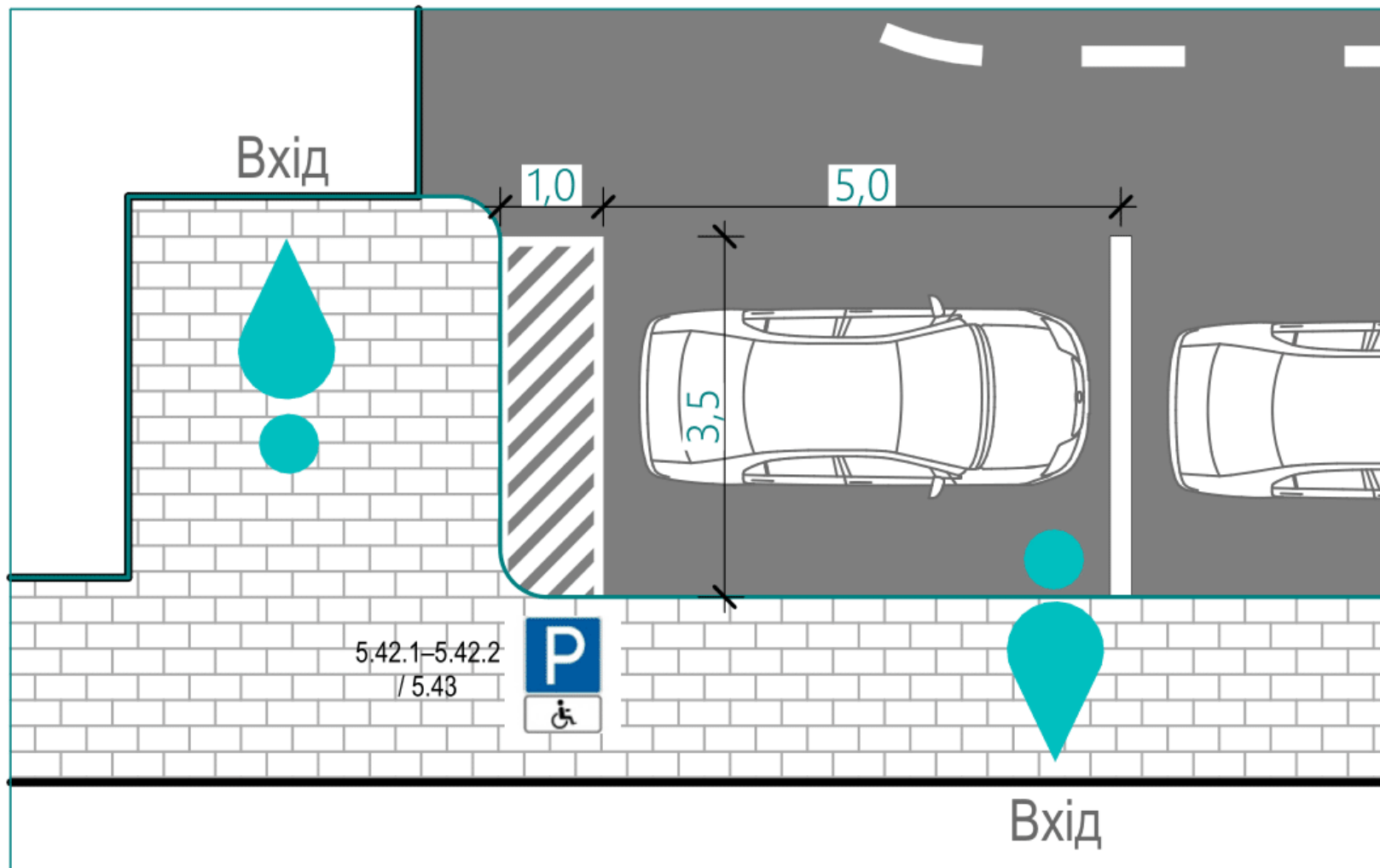
Рис. 11 Схема влаштування паркомісць.
