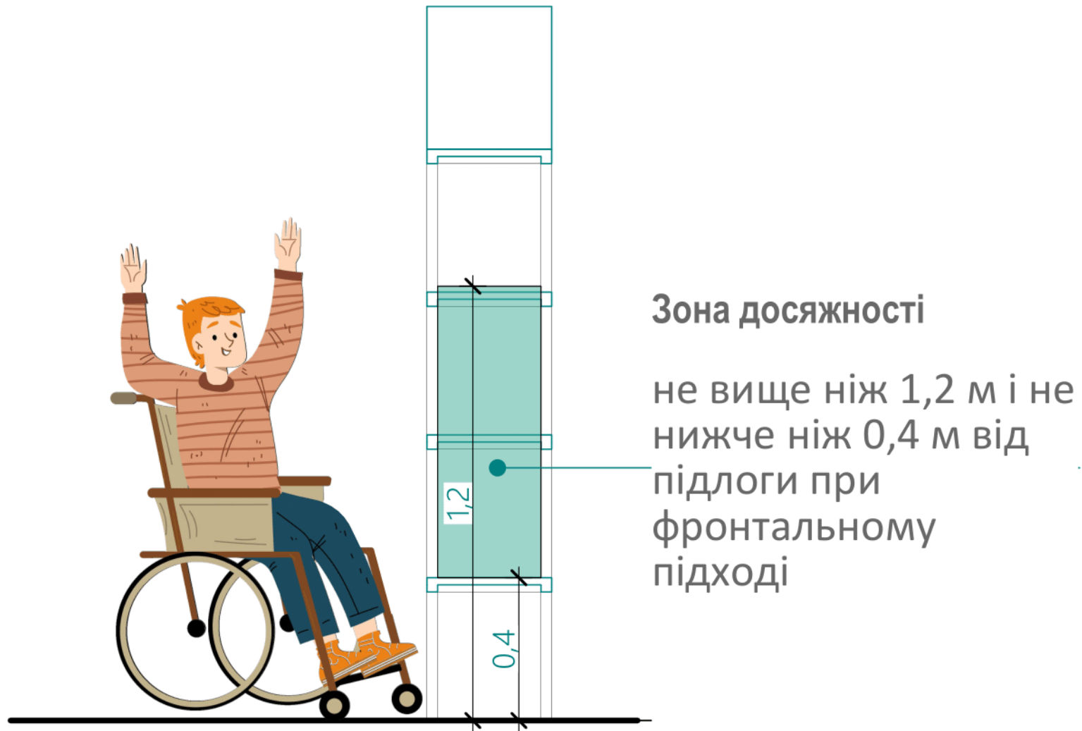
Рис. 19 Схема обладнання торгових площ при боковому підході.
