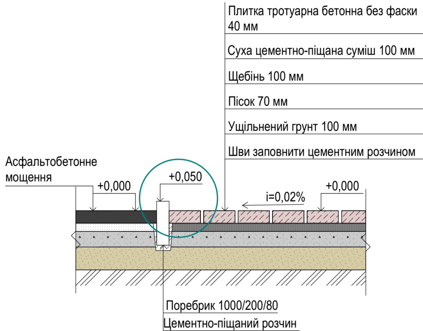
Рис. 4 Вузол влаштування мощення пішохідного шляху.
