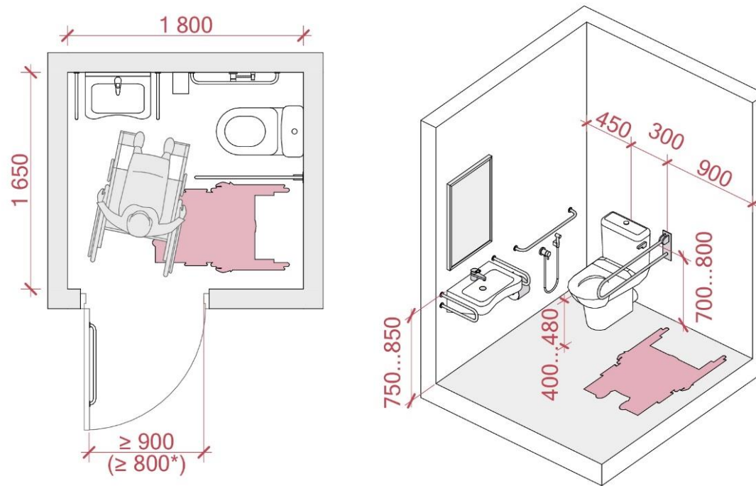
Рис. 29 Орієнтовна схема облаштування універсального санітарного приміщення в мінімальних параметрах.
