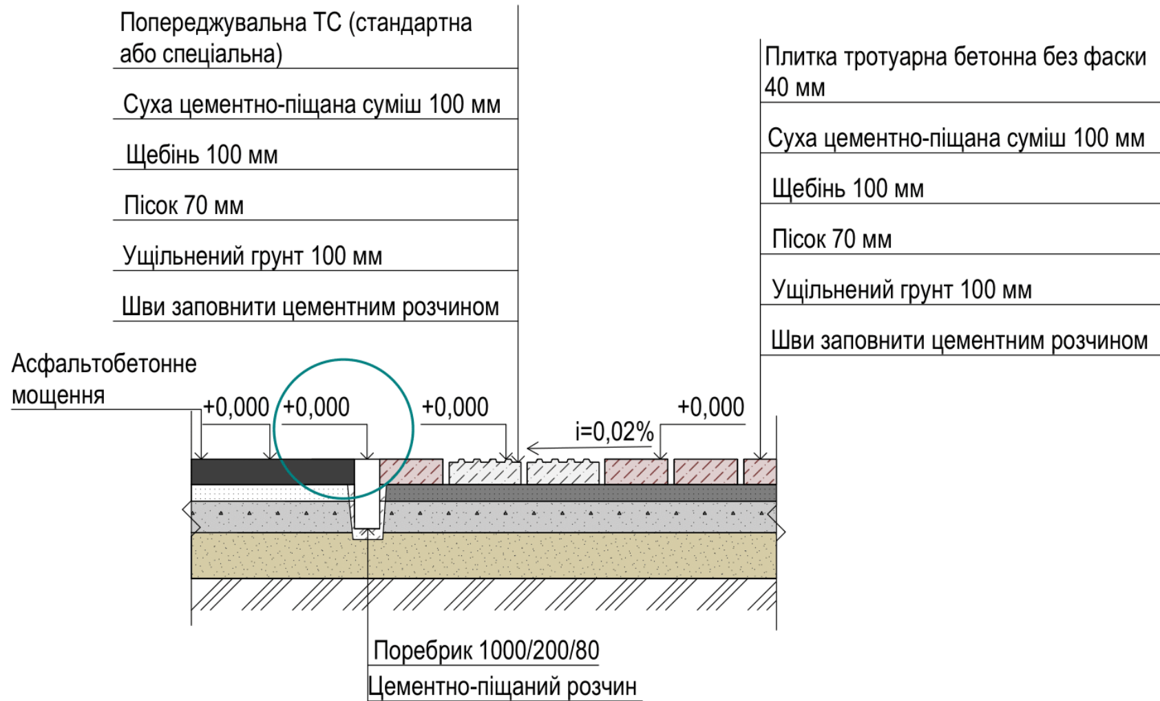
Рис. 3 Вузол влаштування мощення у місці облаштування пішохідного переходу.
