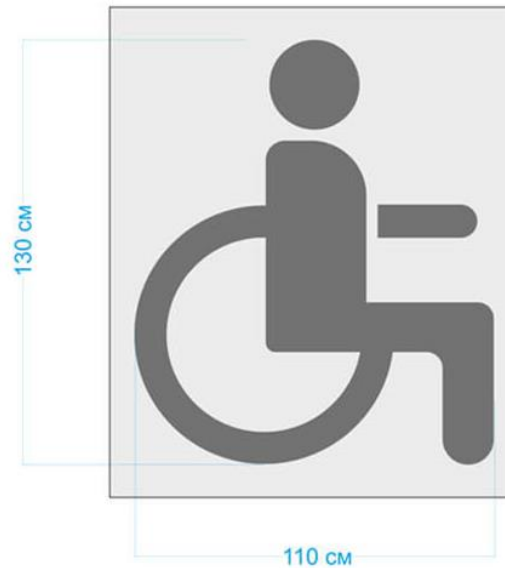
Рис. 12 Трафарет міжнародного символу доступності.
