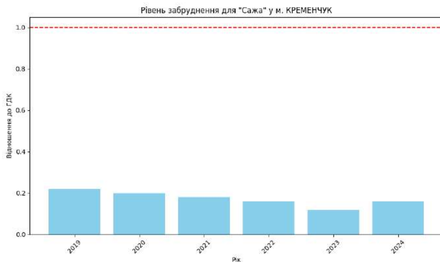
Рис. 2.14 – Сажа
