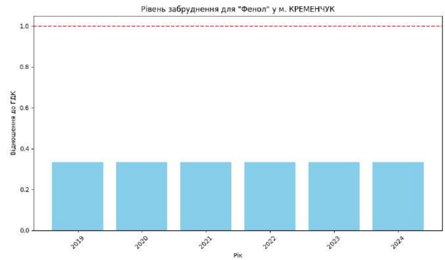
Рис. 2.9 – Фенол
