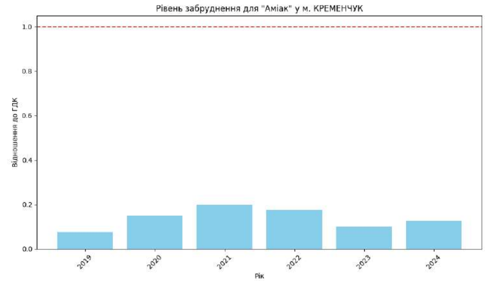
Рис. 2.12 – Аміак
