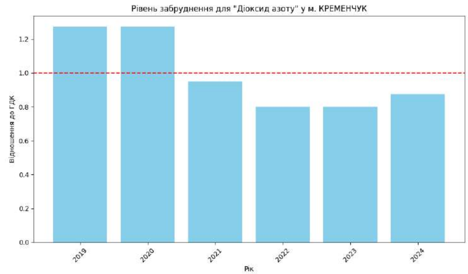
Рис. 2.8 – Діоксид азоту
