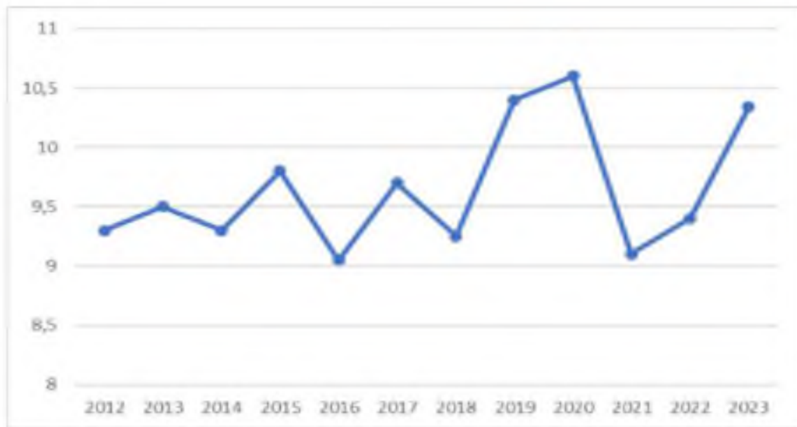
Рис. 4. Хід середньорічної температури повітря на території Полтавської області за період 2012-2023 роки
