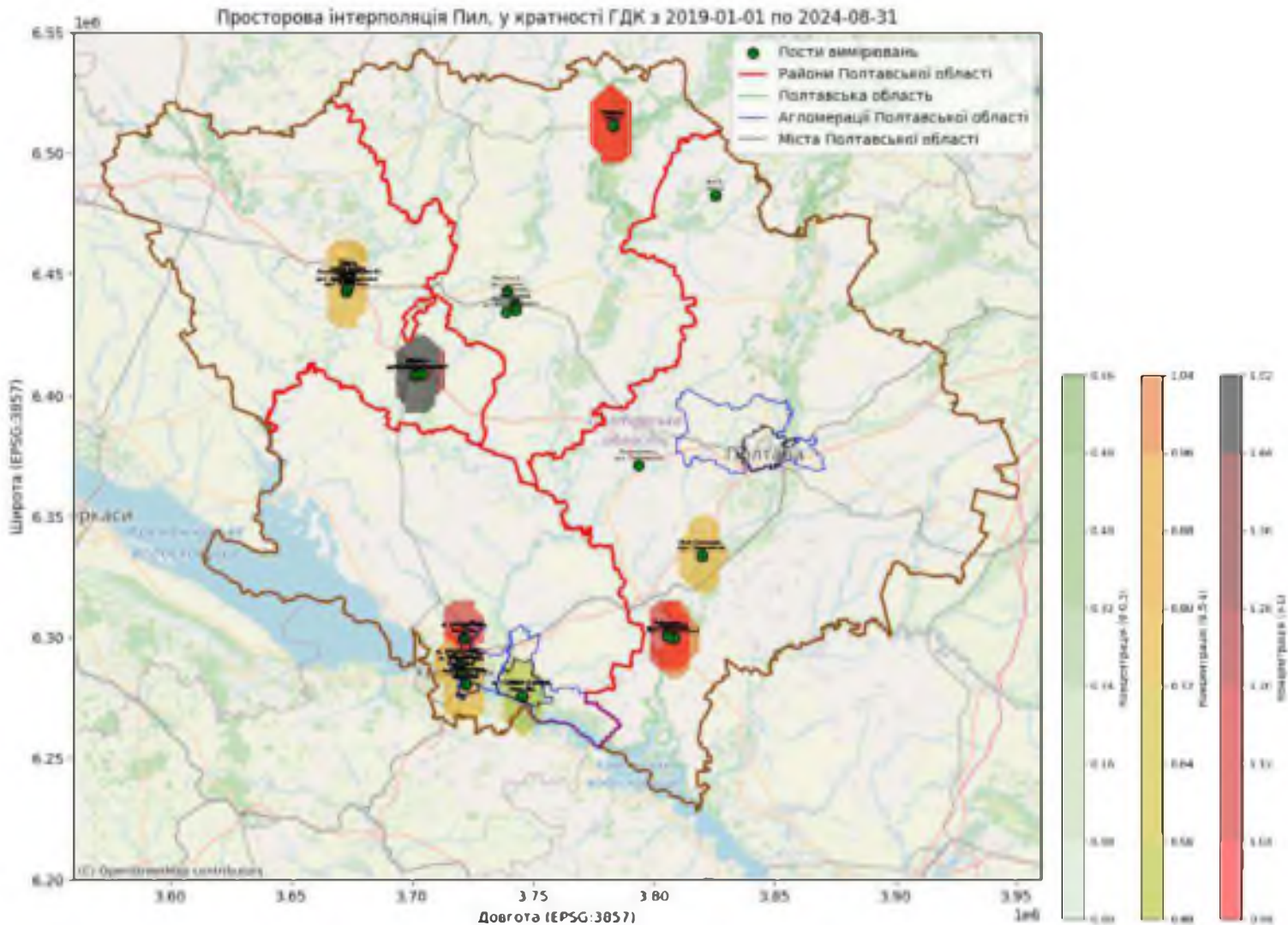
Рис. 3.2 – Просторовий розподіл концентрації пилю в зоні «Полтавська» за період з 2019 по 2024
