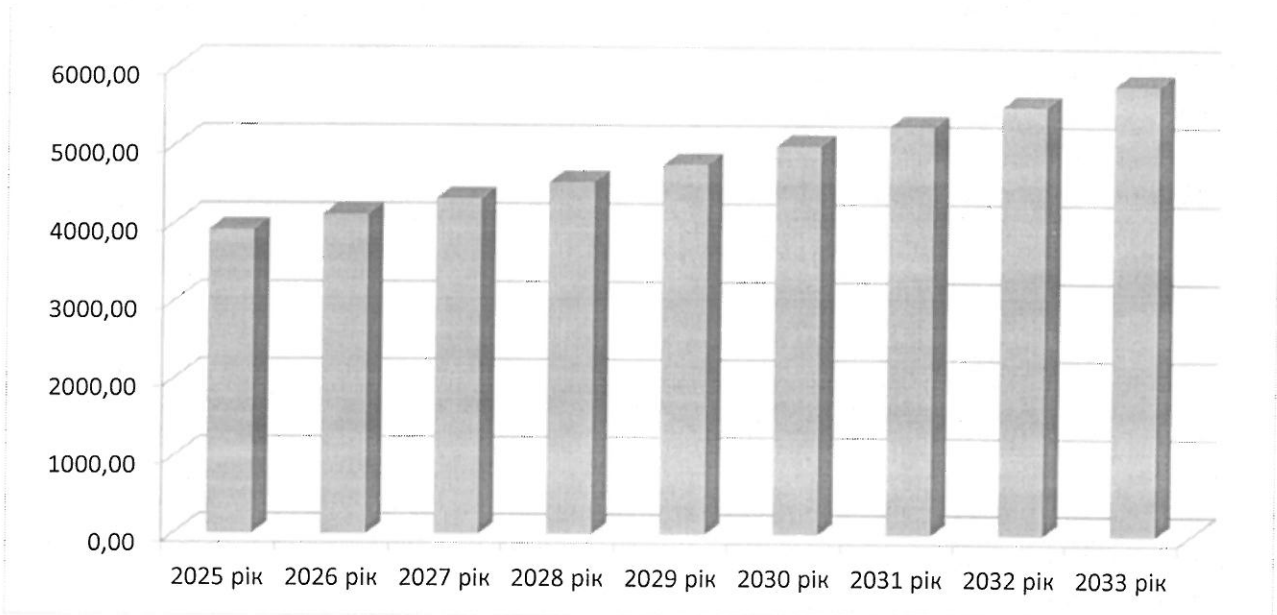
Рис. 5.2 – Прогноз утворення загального обсягу відпрацьованих нафтопродуктів з урахуванням тенденції динаміки 2014-2022 років, т
