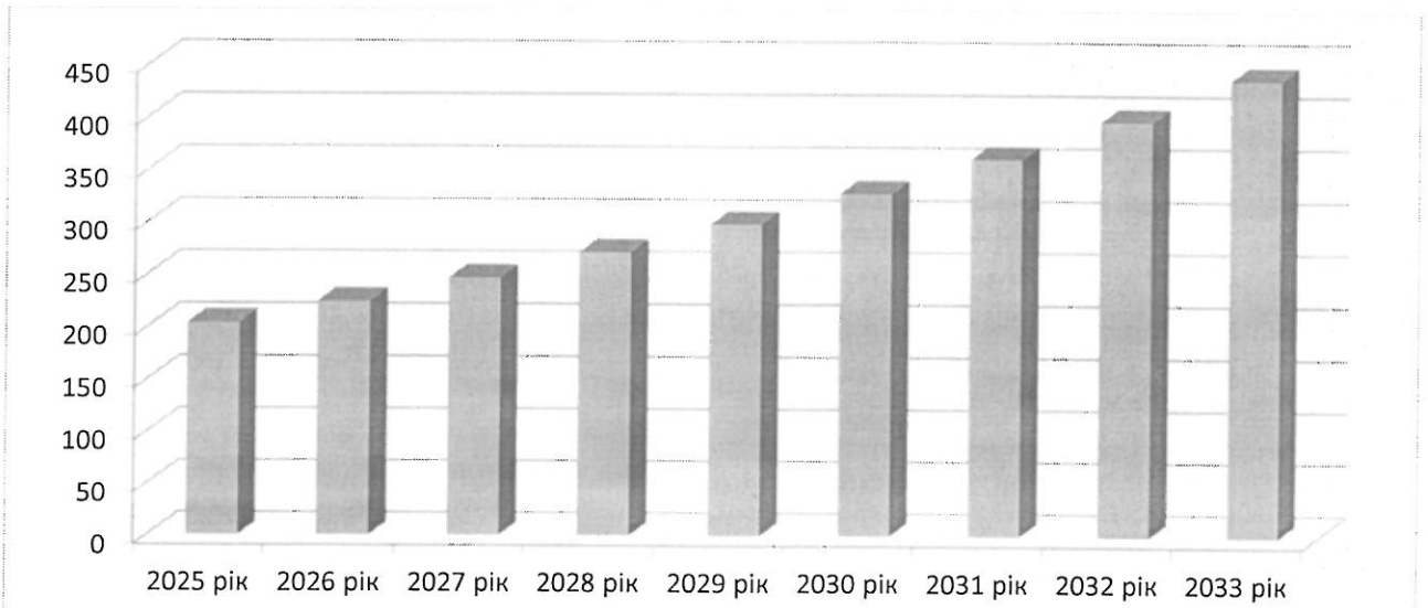
Рис. 5.1 – Прогноз утворення загального обсягу медичних відходів (за динамікою відходів від медичної допомоги та біологічні з урахуванням тенденції динаміки 2014-2023 років), т
