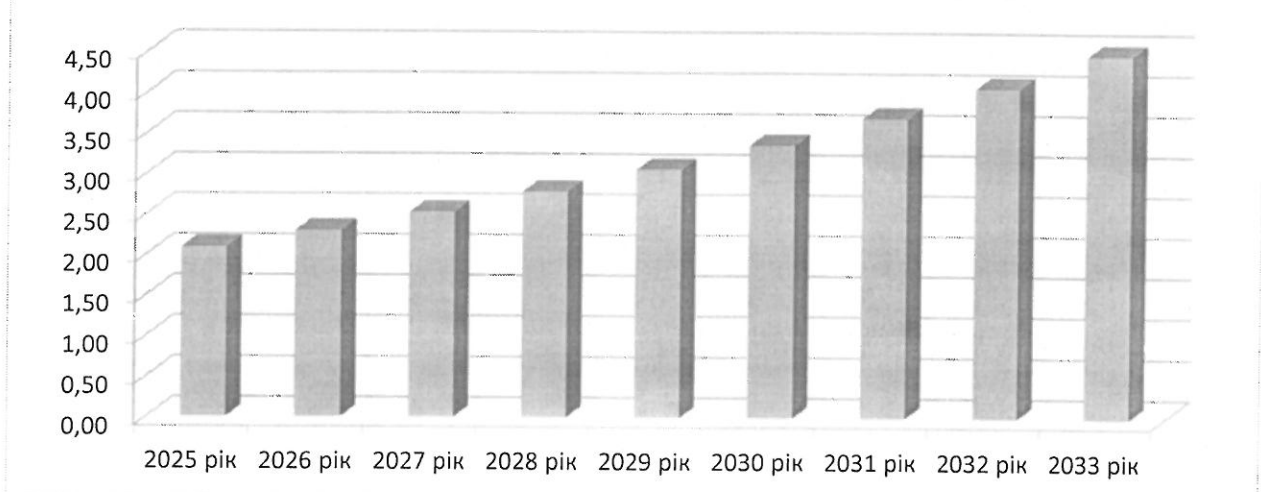
Рис. 5.3 – Прогноз утворення загального обсягу непридатних транспортних засобів з урахуванням тенденції динаміки 2014-2022 років, т
